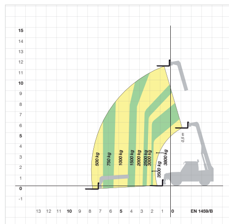
P 38.12 / PLUS MIT LASTGABELN AUF RÄDERN
