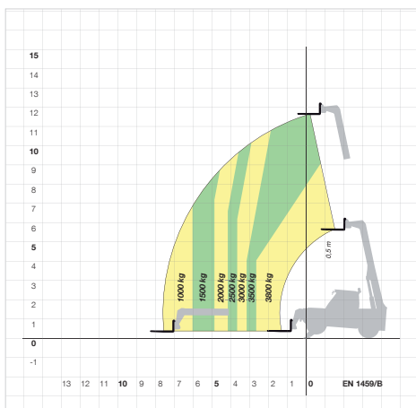
P 38.12 / PLUS MIT LASTGABELN AUF ABSTÜTZUNGEN
