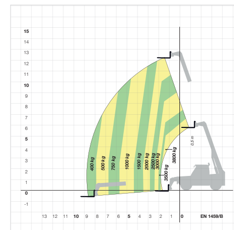
P 38.13 MIT LASTGABELN AUF RÄDERN
