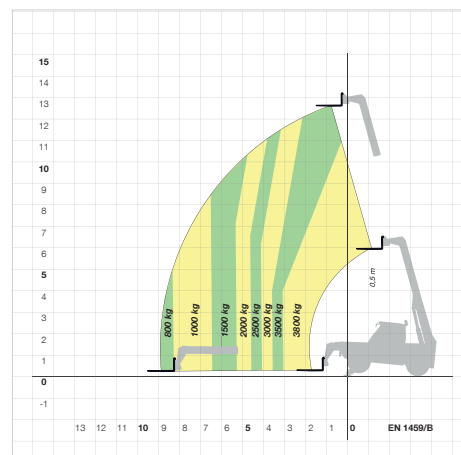
P 38.13 MIT LASTGABELN AUF ABSTÜTZUNGEN
